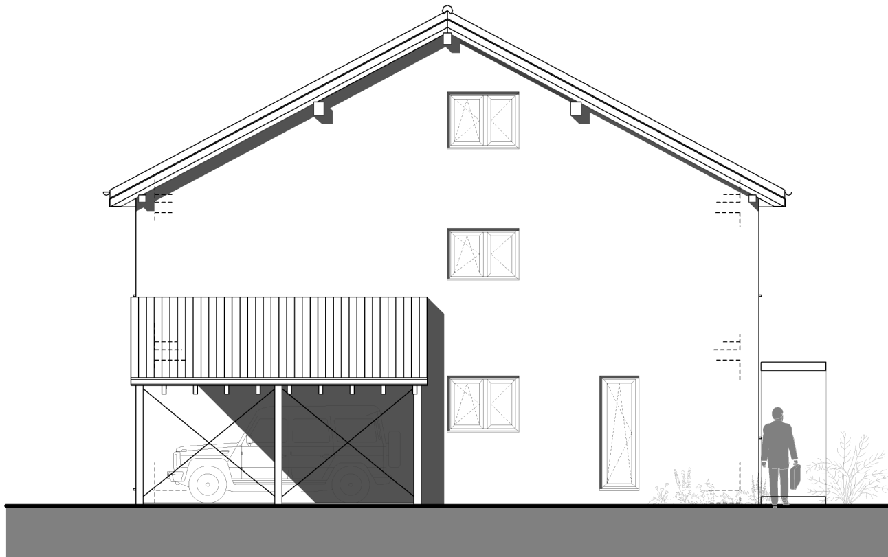
Seitenansicht
